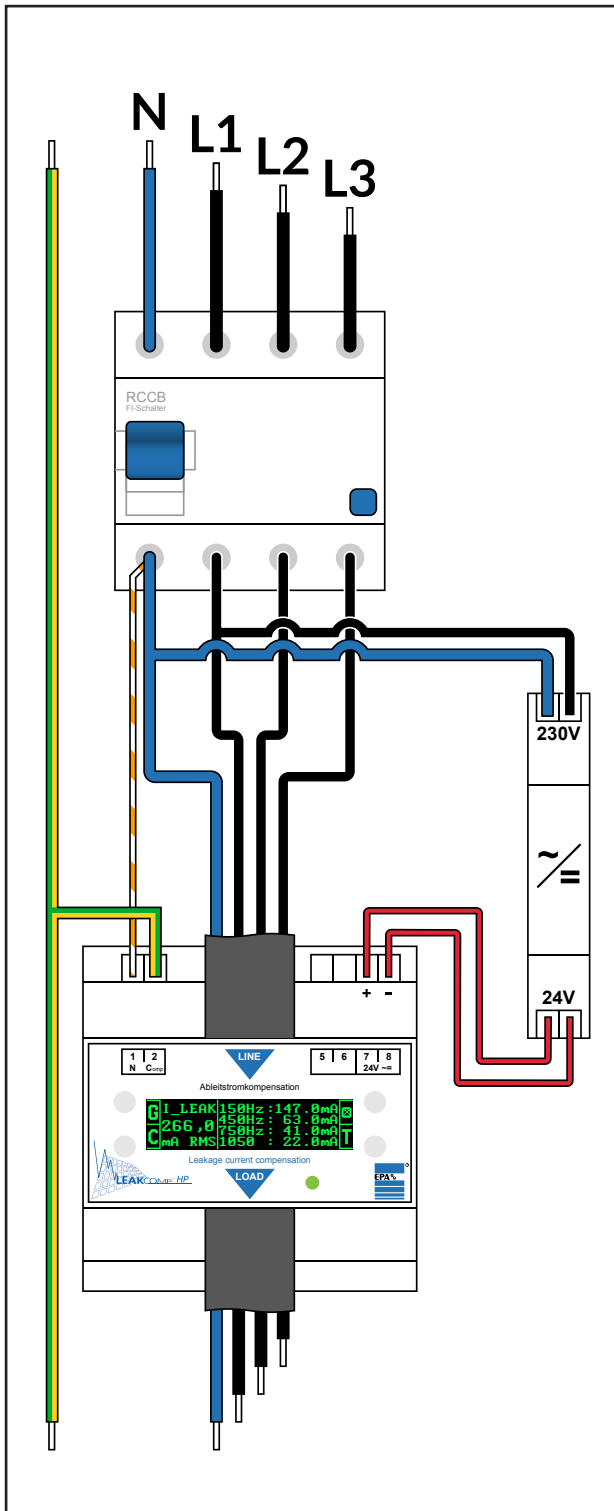
Anschluss-Schema mit Neutralleiter Wiring diagram with neutral conductor
