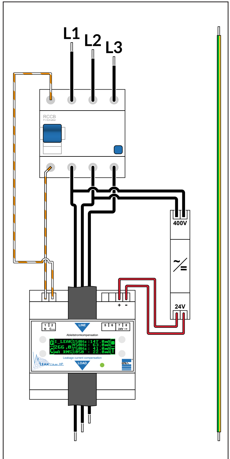
Anschluss-Schema ohne Neutralleiter Wiring diagram without neutral conductor
