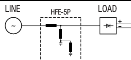
Electrisch schema
