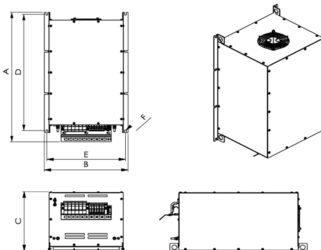
Afmetingen
